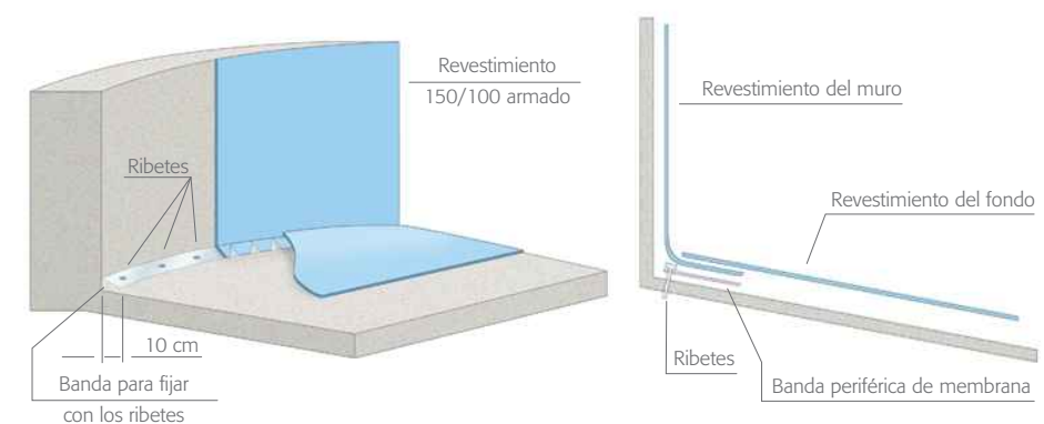
Figura 16: Fondo plano sobre pared curva
