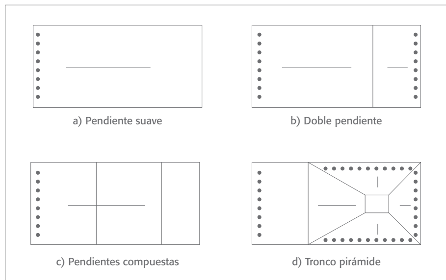
Figura 14: Fijación mecánica en las pendientes
