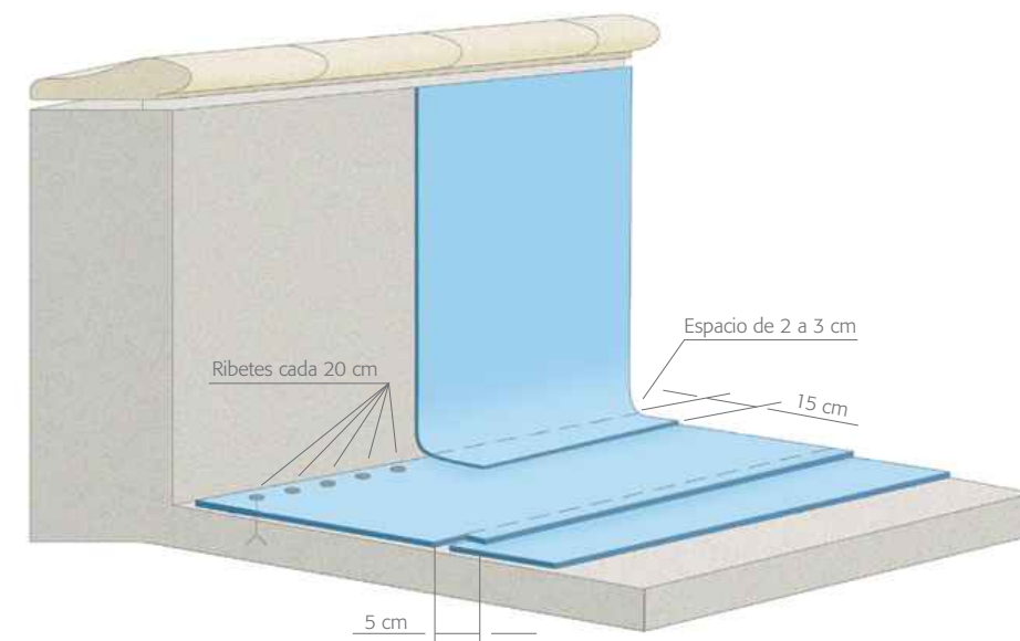
Figura 15: Soldadura pared / fondo (pared rectilínea)
