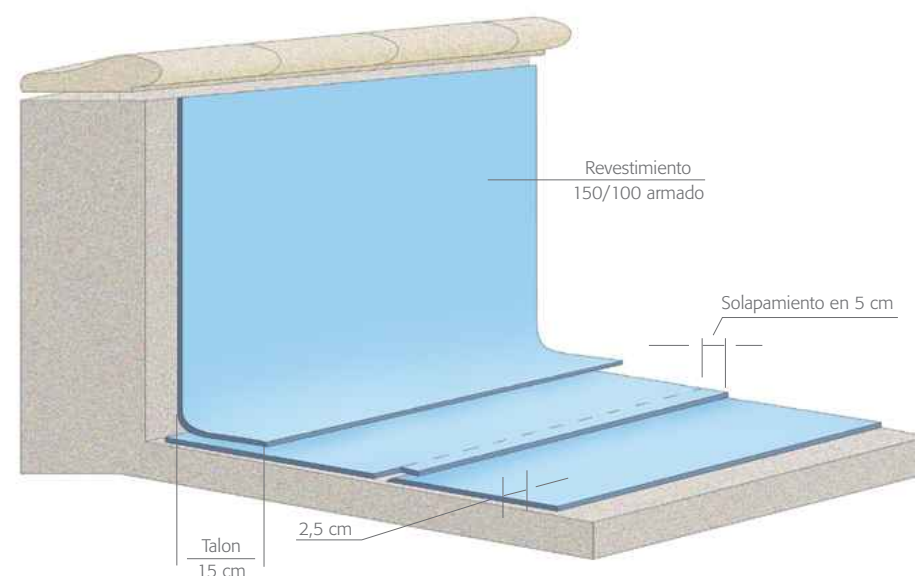
Figura 10: Fondo plano no fijado
